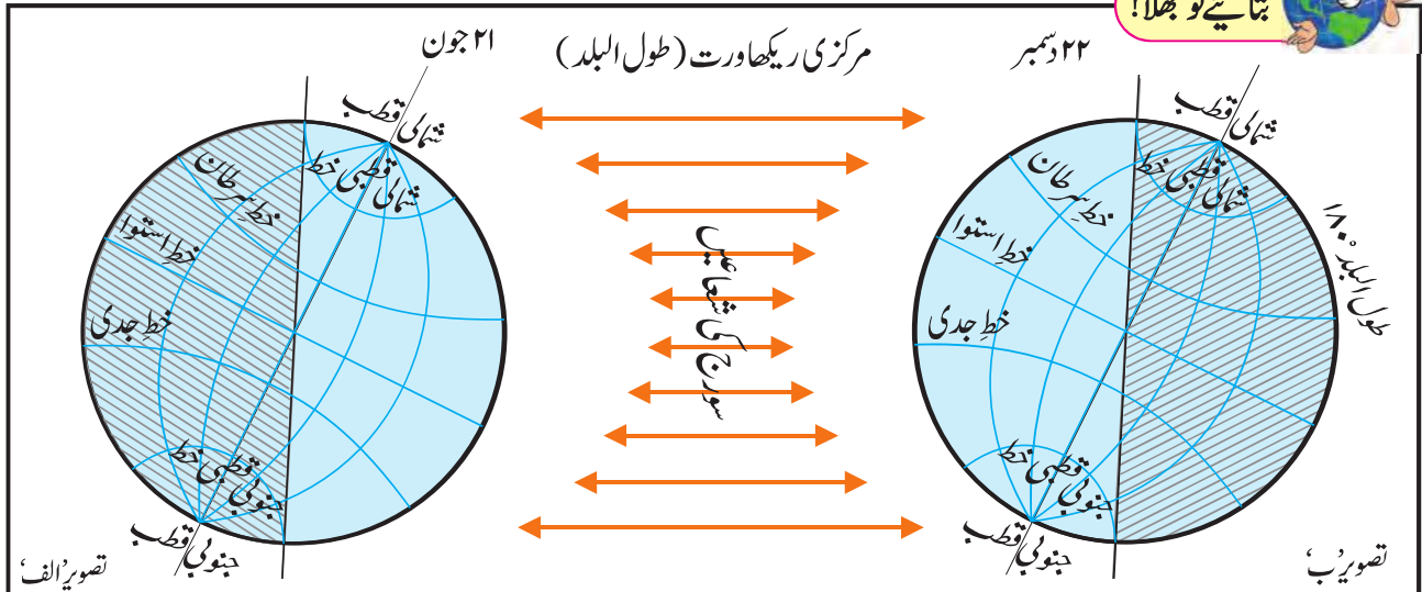
شکل ۸ء۴: محوری جھکاؤ کے ساتھ زمین کی ۲۱ جون اور ۲۲ دسمبر کو سورج کے مقابل حالت
