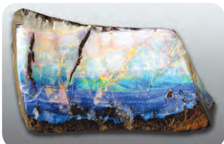
Fig. 5.8 : Opal
