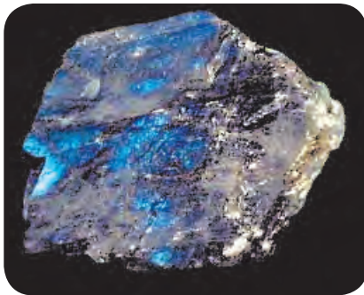
Fig. 5.13 : Labradorite
