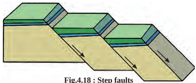
Fig.4.18 : Step faults
