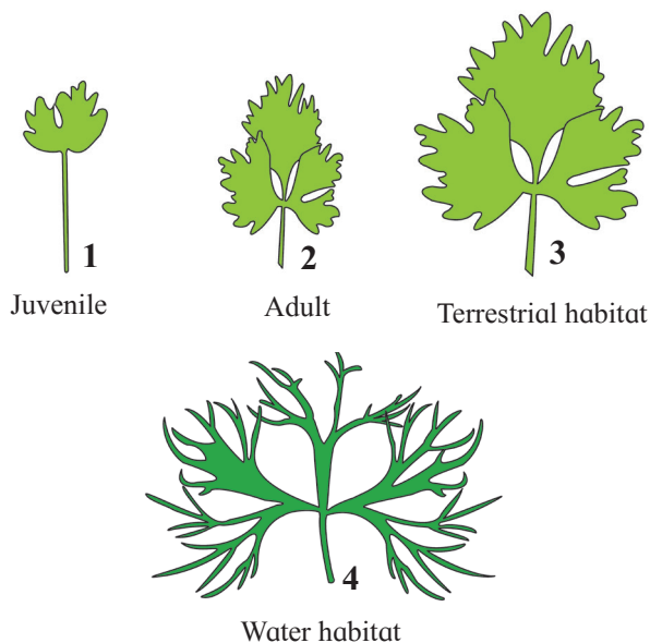
Fig. 7.8 Heterophylly
