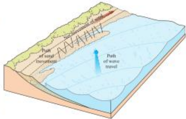
Fig. 3.9 : Longshore drift
