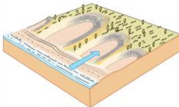
Fig. 3.28 : Parabolic dunes
