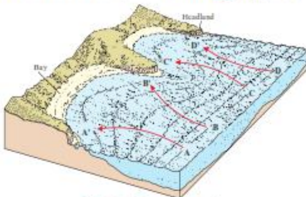
Fig. 3.8 : Wave refraction
