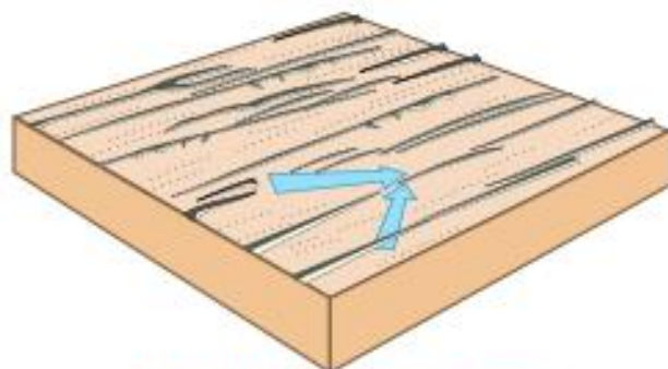
Fig. 3.26 : Linear or Self dunes
