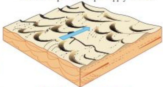
Fig. 3.24 : Transverse dunes
