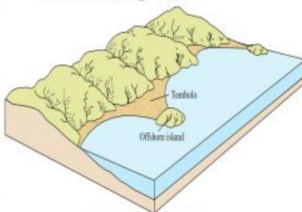
Fig. 3.14 : Tombolo
