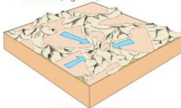
Fig. 3.27 : Star dunes
