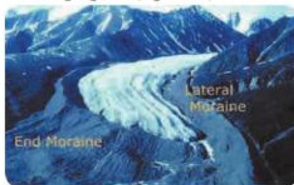
Fig. 3.34 : Glacial moraines
