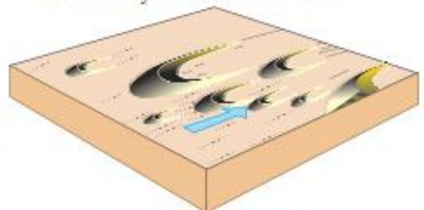
Fig. 3.25 : Barchan dunes
