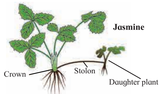
Fig. 9.24 Stolon
