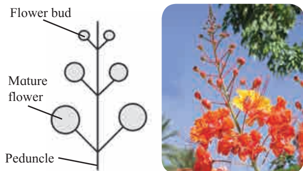
Fig. 9.39 Racemose
