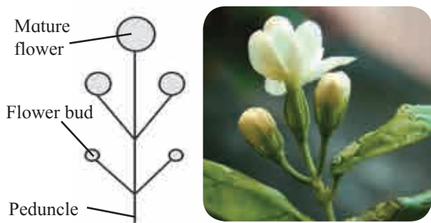
Fig. 9.40 Cymose
