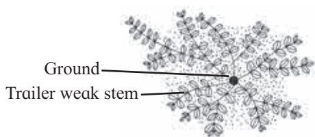
Fig. 9.22 Euphorbia trailer
