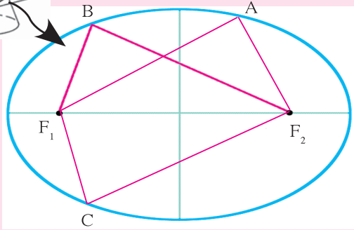
1.3: بیضوی مدار
